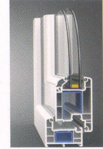
Casement Door
